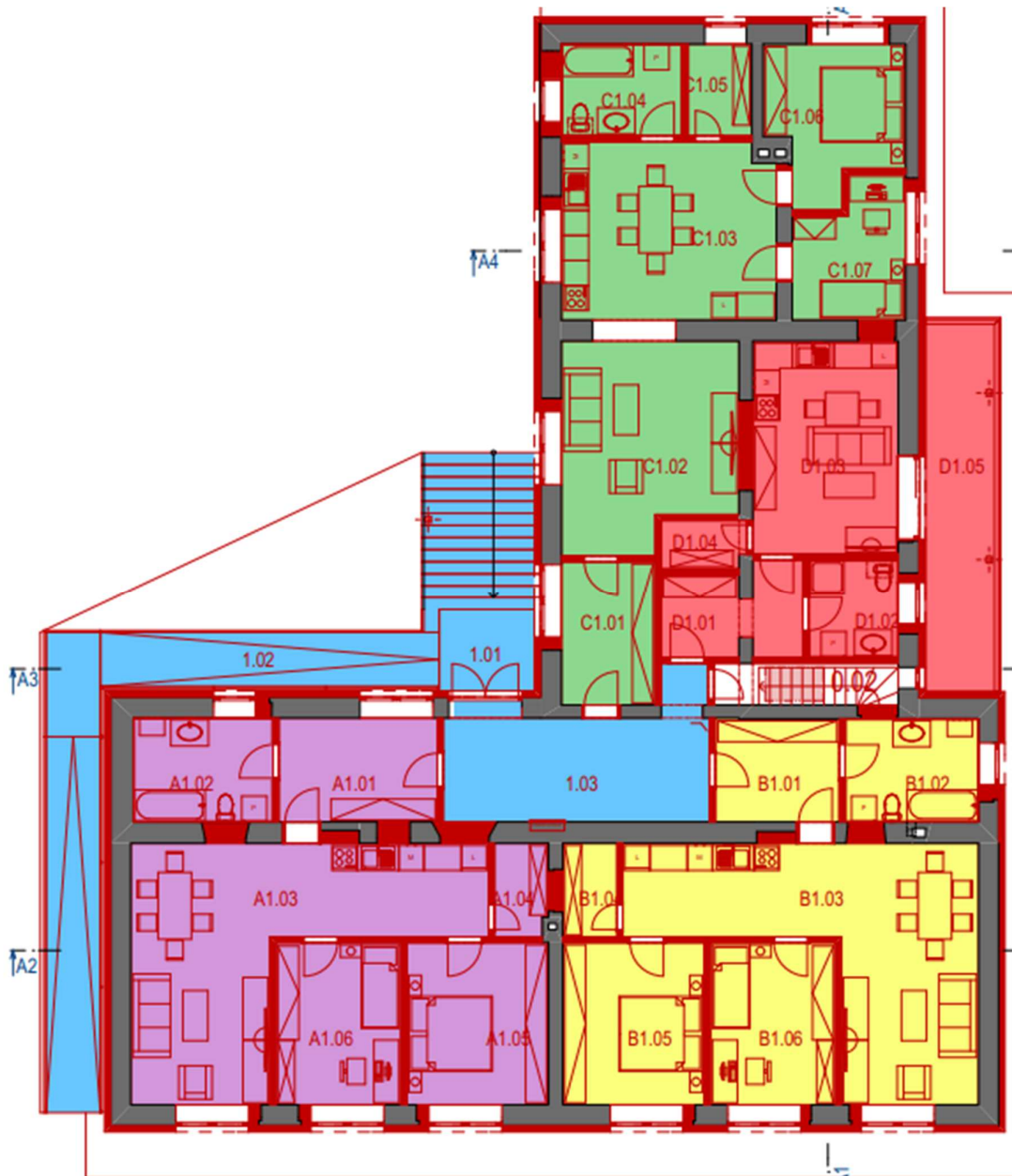
Príloha č. 6: Pôdorys bytov
